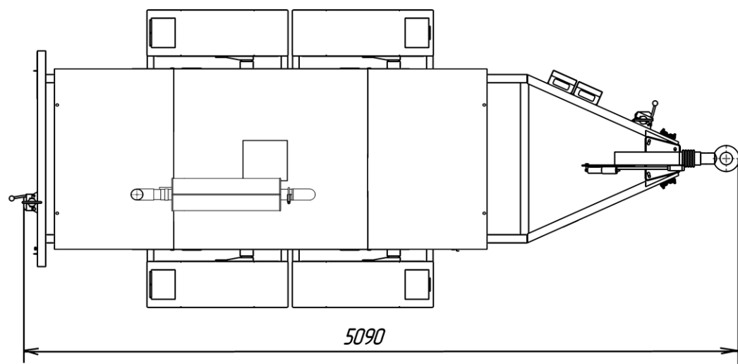
Рисунок В.2 Станция компрессорная передвижная дизельная ЗИФ-ПВ22,5/1,03 (АРМ9-36-03) Исполнение на прицепе. Габаритный чертеж
