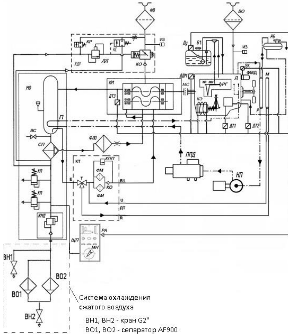
Рисунок В.19 - Схема комбинированная функциональная с системой охлаждения сжатого воздуха
