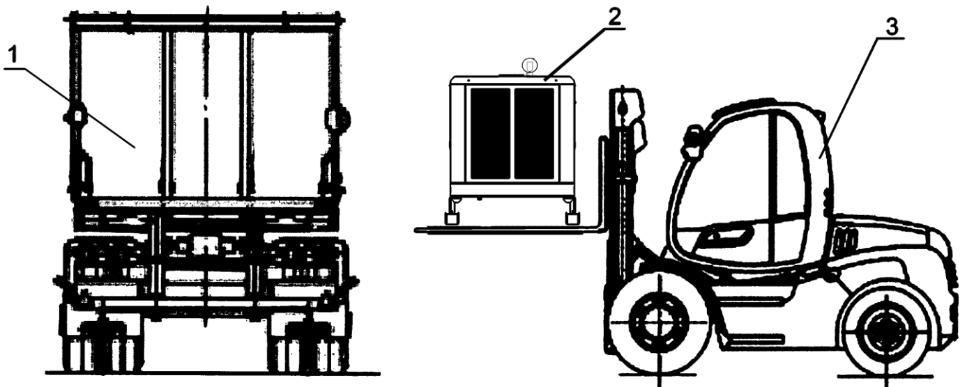
1 – кузов транспортного средства; 2 - компрессорная станция; 3 – вилочный погрузчик;
